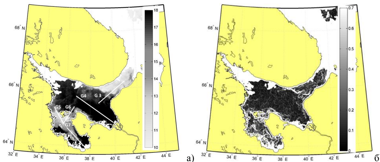
Рис. 4.4 Карта ТПО (а) и ее горизонтального градиента (б), рассчитанные по данным MODIS Terra от 4.08.2010 г. На карту ТПО нанесены разрезы (G3-G7), с которых снимались характеристики фронтальных разделов во фронтальных зонах.
