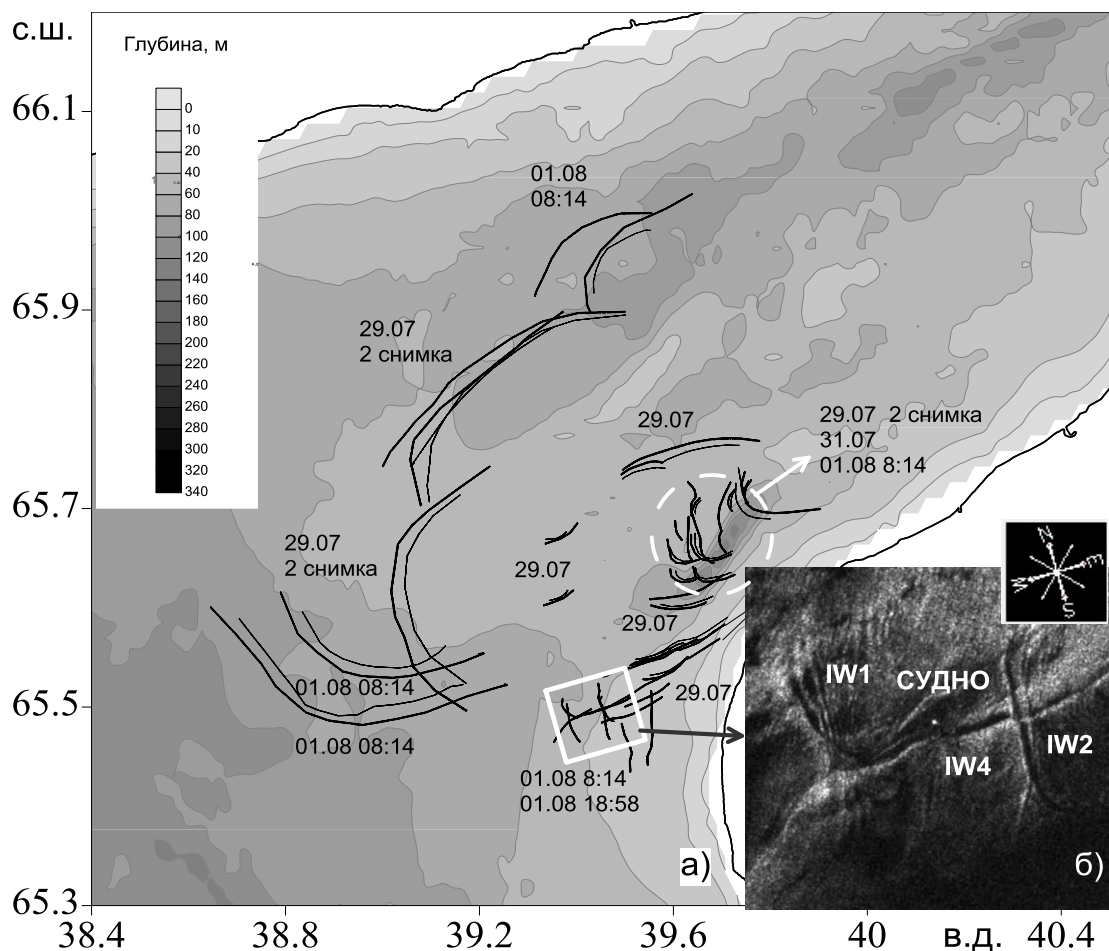
Рис. 3.10. Обобщенная схема поверхностных проявлений ВВ по пяти РЛ-изображениям района экспедиционных работ (а). Толстые линии обозначают положение гребня лидирующих волн в пакетах, тонкие – положение гребня третьей волны в пакете. На врезке (б) представлен
