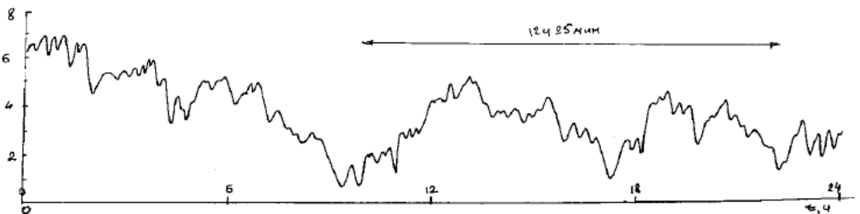
Рис.1.7 Запись внутренних волн распределенным датчиком температуры, сделанная на суточной станции [Серебряный и др., 2009].
