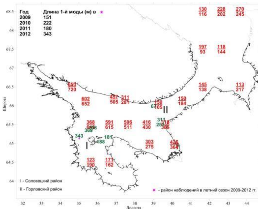
Рис. 3.17. Длина волны (в метрах) первой моды периода 12 мин по климатическим данным (красным: верхняя цифра – июнь, нижняя – август), а также по результатам полигонных измерений 2012 г (зеленые цифры) и в районе, обозначенном звездочкой (в табличной врезке).
