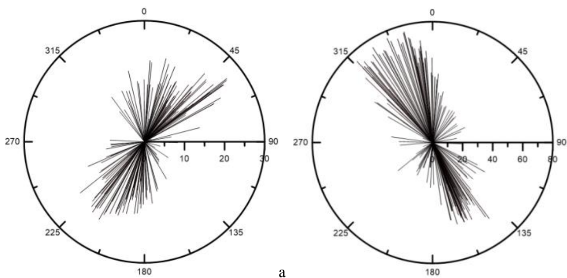
Рис. 2.14. Векторные диаграммы распределения скоростей течений по данным, полученным с 08:23 по 20:47 24 июля 2012 г. на полигоне № 4 (а) и с 0:00 по 12:24 23 июля 2012 г. на
