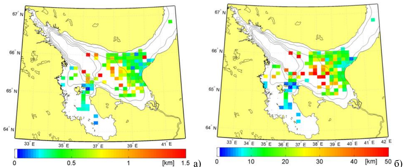
Рис. 3.16. Пространственная изменчивость проявлений ВВ за теплый период 2007, 2009-2013 гг. (а), длины лидирующей волны в пакете (а), длина гребня (б) по данным РЛИ за 2007, 2010, 2012-2013 гг.
