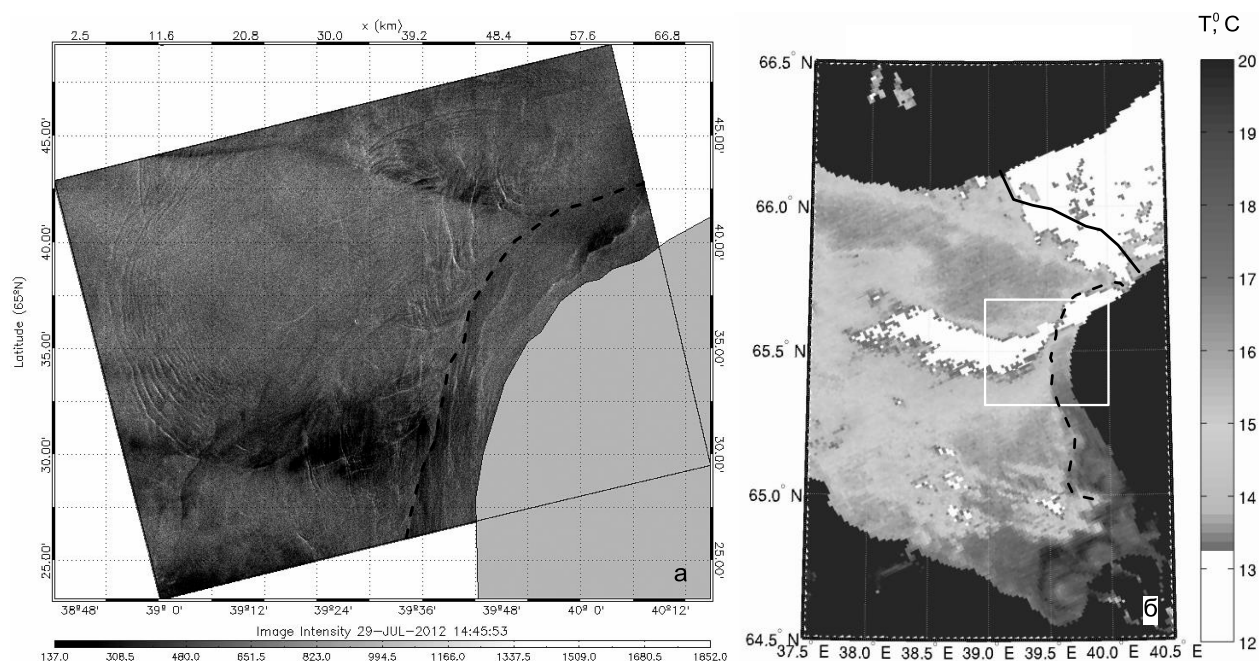
Рис. 3.8 Фрагмент РЛ-снимка RADARSAT-2 от 29.07.2012 (а) и поле температуры поверхности моря по данным MODIS TERRA от 30.07.2012 (б). Прямоугольником на фрагменте (б) показан район (а). Пунктиром на изображениях обозначено положение стокового фронта по данным поверхностных проявлений, сплошной линией – реконструкция положения структурного фронта по данным контактных наблюдений 2012 г и литературным источникам. © CSA © NASA.
