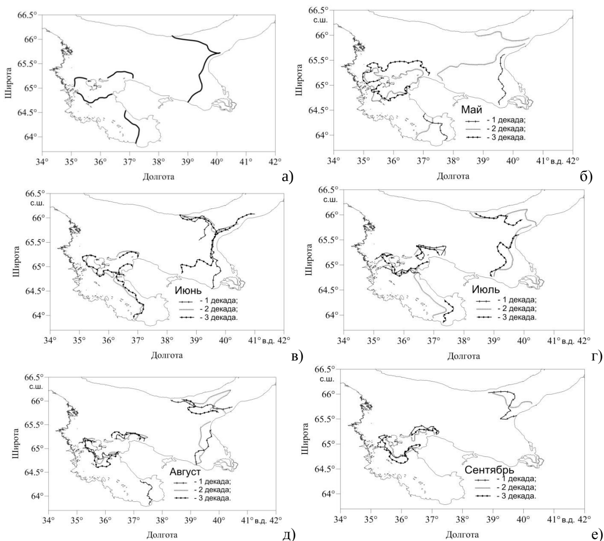
Рис. 4.6 Схемы расположения основных фронтов по данным спутниковых наблюдений в Белом море за теплый сезон (а) и с мая по сентябрь (б-е) с разделением по декадам за 2010 год.
