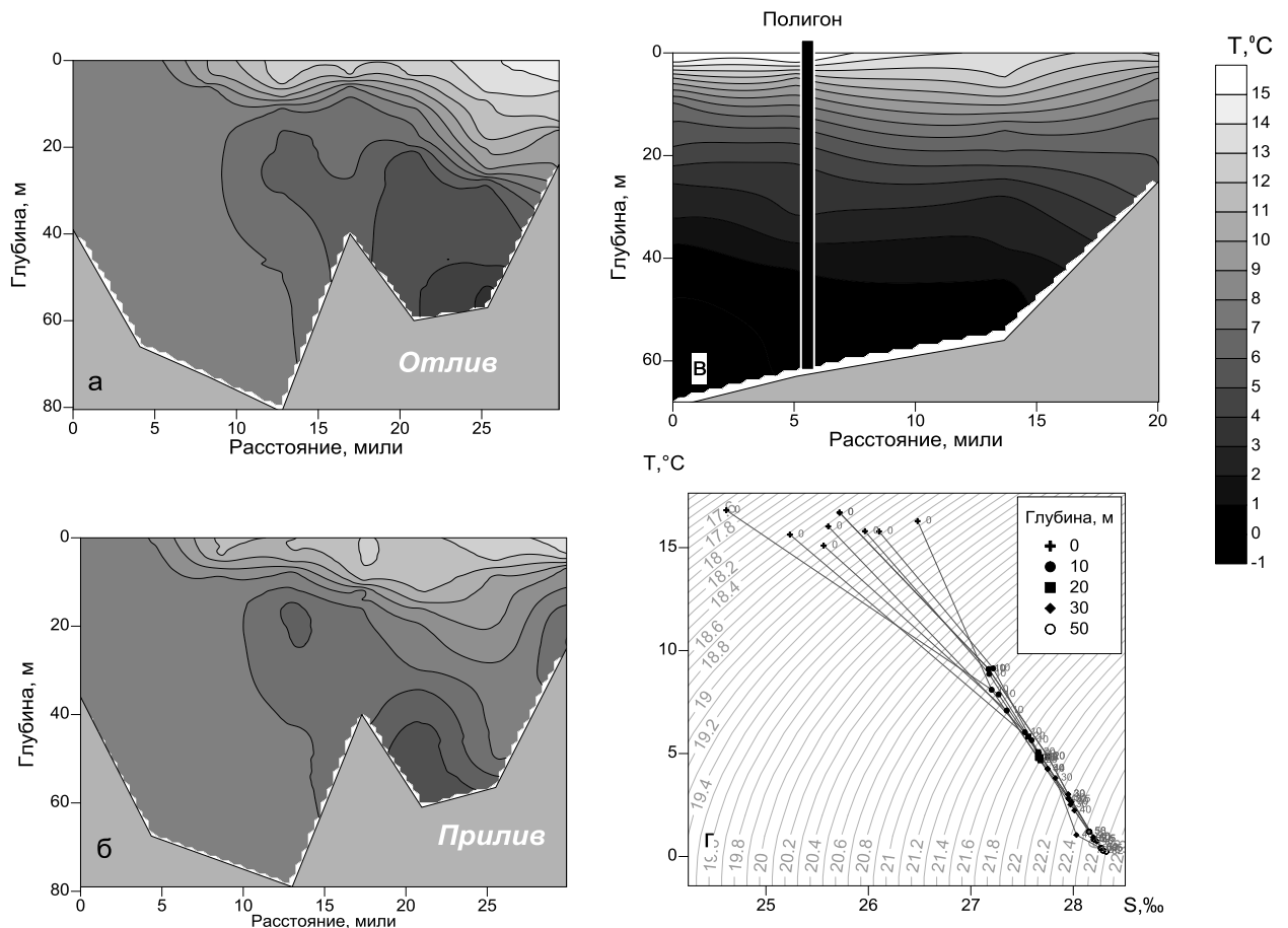
Рис. 3.7. Распределение температуры на гидрологических разрезах, выполненных поперек Горла Белого моря 30.07.2012 (а) и 31.07.2012 (б) в разные фазы приливного цикла, на разрезе вдоль Зимнего берега 31.07.2012 (в) и T, S – кривые по данным наблюдений на полигоне 31.07.2012 (г). Горизонты наблюдений обозначены на рисунке (г) значками, соответствующие им глубины приведены в верхней правой части.
