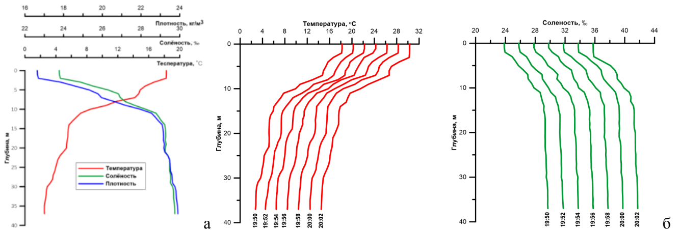
Рис. 2.19. Характерные профили температуры, солёности и условной плотности для полигона №14 июль 2014 года (а) и серии профилей температуры и солёности, записанные 26 июля 2014 года (б)
