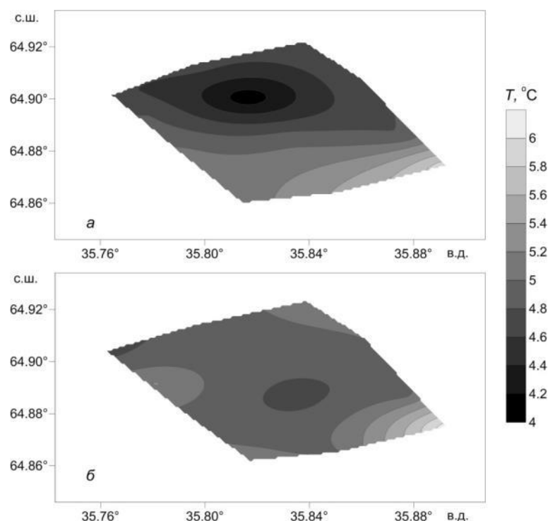
Рис. 4.2. Распределение температуры на горизонте 10 метров по данным микрополигонных океанографических съемок на полигоне № 9, выполнявшихся в прилив (а) и отлив (б) 24 июня 2009 года.
