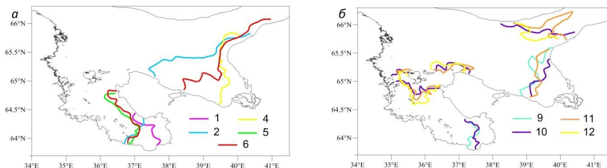
Рис. 4.8 . Изменчивость положения фронтальных линий по спутниковым данным о ТПМ: а – Двинский и Онежский фронты в мае и июне; б – все фронты в конце июля и в августе. Цифры на линиях указывают номер декады, начиная с первой декады мая.
