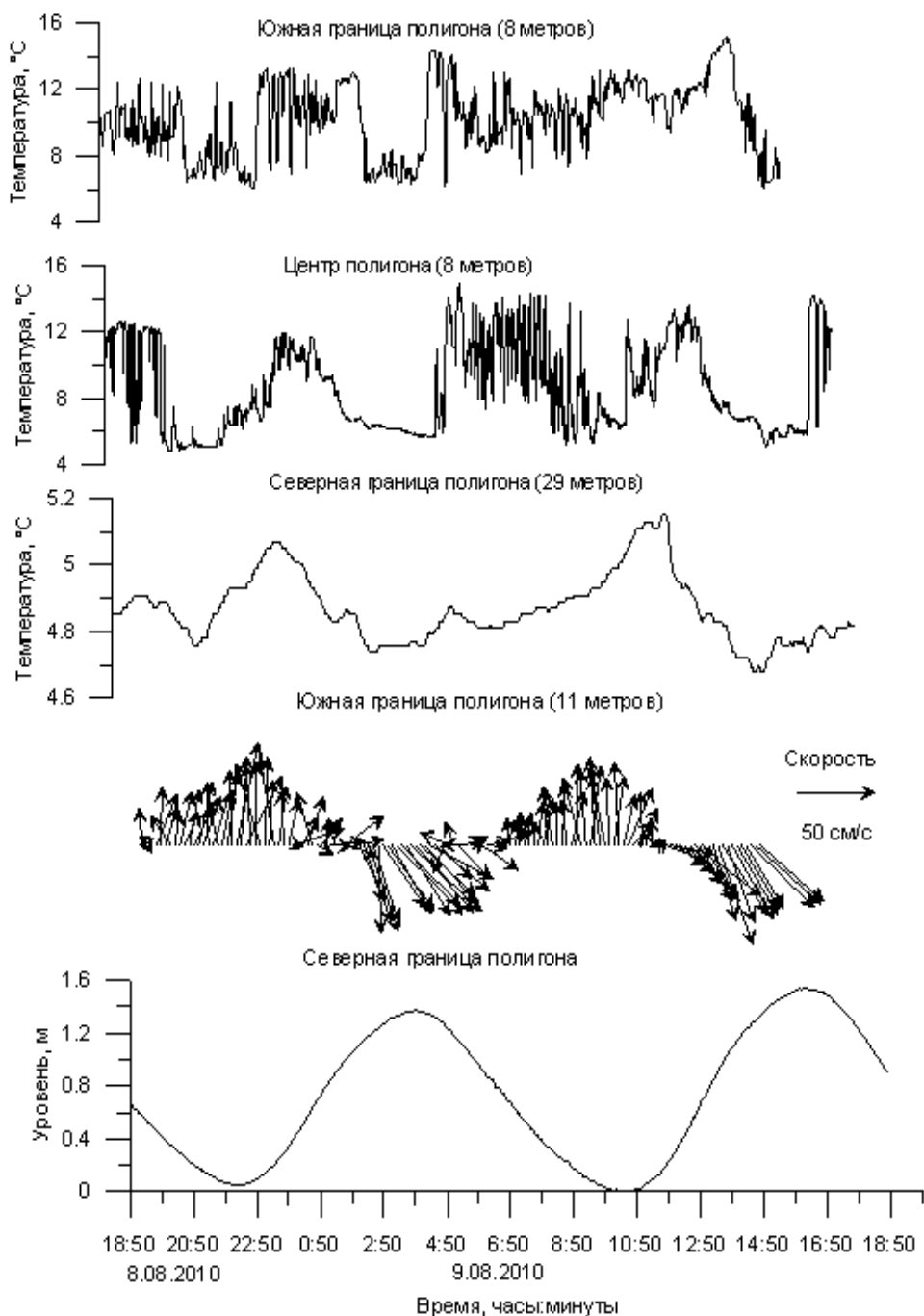
Рис. 3.1 Временная изменчивость температуры по данным наблюдений с 18:50 8 августа до 19:20 9 августа 2010 года на южной, центральной и северной буйковых станциях, скорости и направления течения на южной буйковой станции, колебания уровня по показаниям датчика давления на северной буйковой станции.
