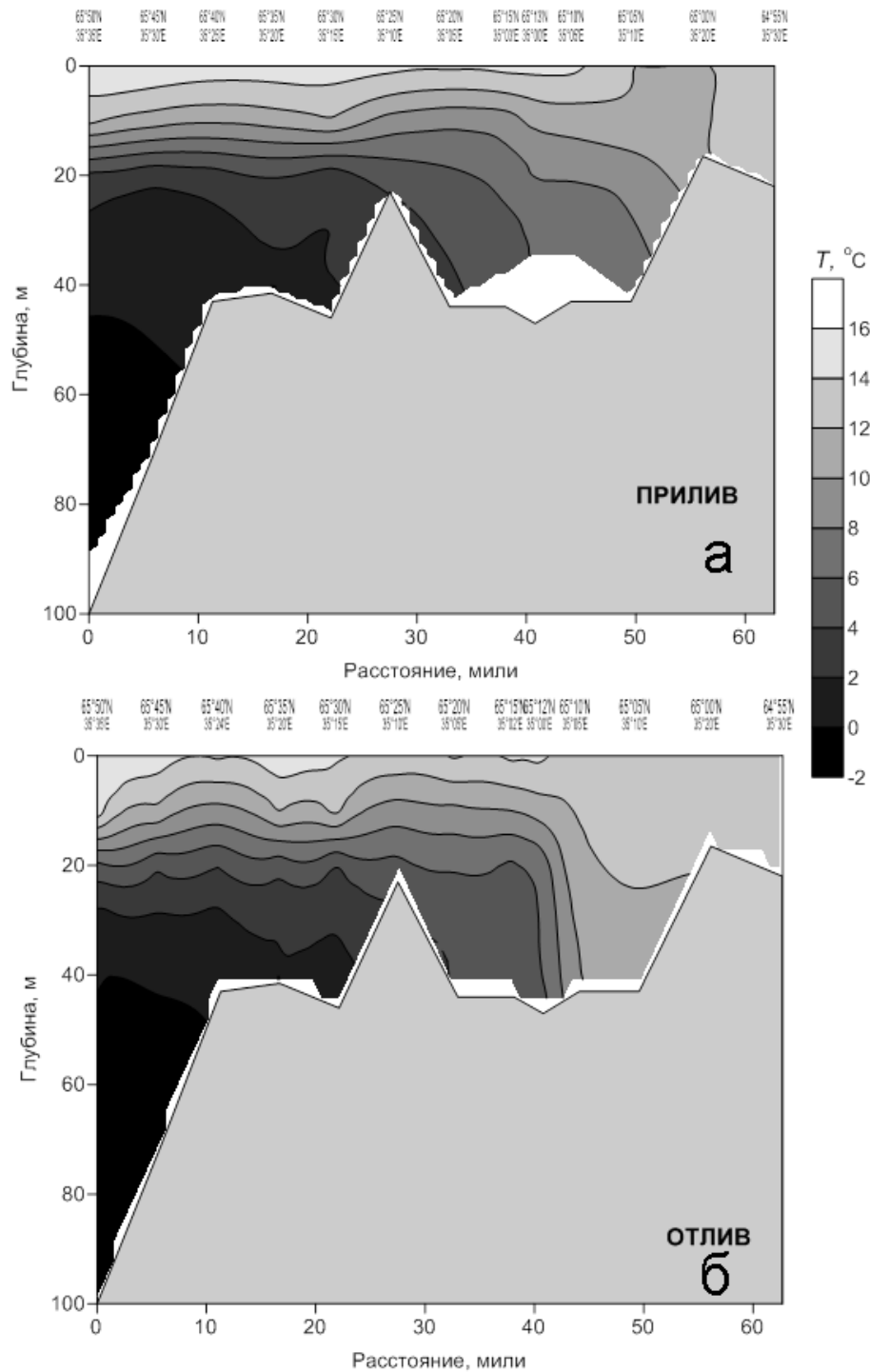
Рис. 4.13. Распределение температуры на гидрологических разрезах, выполненных поперек шельфа от котловины Белого моря к Онежскому заливу 17.08.2013 (а) и 18-19.08.2013 (б), в разные фазы приливного цикла.
