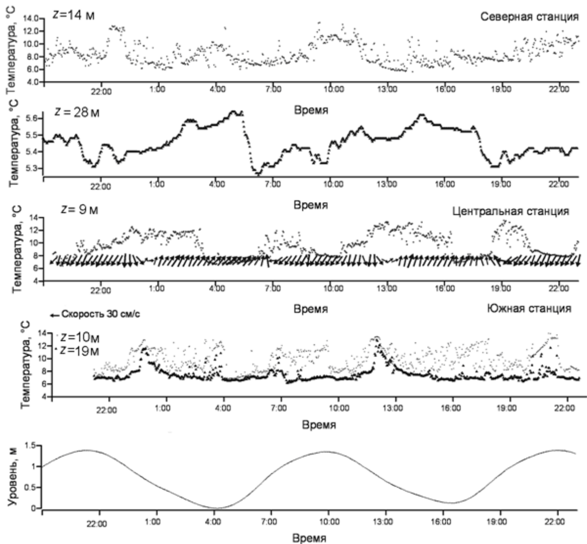
Рис. 2.5. Вариации температуры воды на южной, центральной и северной станциях, скорости и направления течения на центральной станции и колебаний уровня на северной
