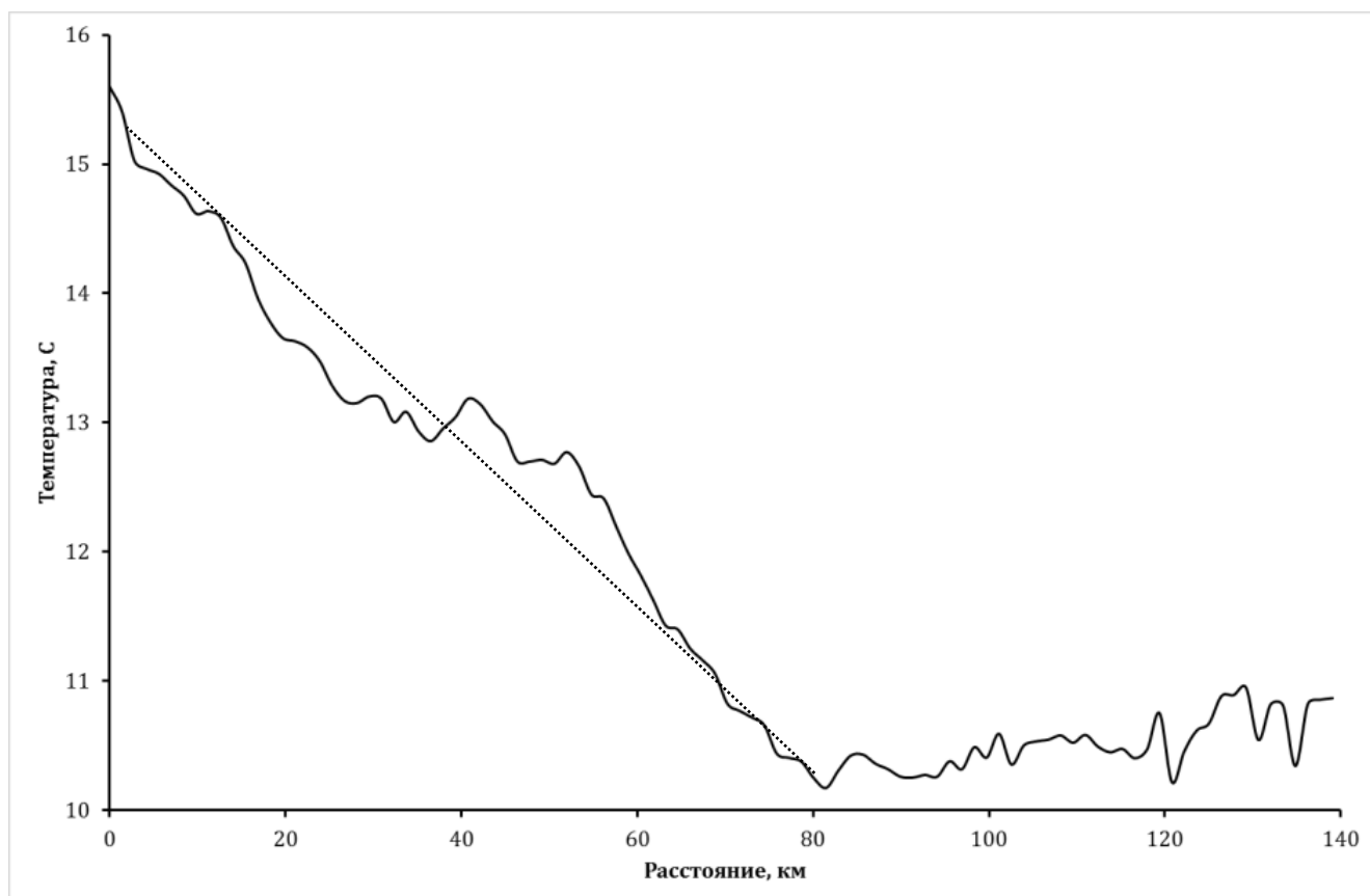
Рис.4.12. Распределение ТПМ на разрезе G4 (от устья до Бассейна) через фронтальную зону реки Северная Двина по данным за третью декаду июня 2010 года.
