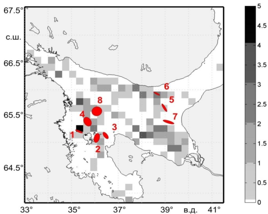
Рис. 5.1. Эллипсы горизонтального турбулентного обмена (обозначены красным) с номерами советующих полигонов, выполненных в июле – августе 2012 года, совмещенные с частотой встречаемости проявлений субмезомасштабных вихревых структур (обозначены серым) по данным РЛИ за 2009-2012 гг. Шкала справа показывает количество вихрей (шт) зарегистрированных в квадрате с заданной площадью.
