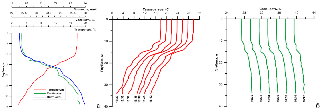
Рис. 2.18. Характерные профили температуры, солёности и условной плотности для полигона №12 август 2013 года (а) и серии профилей температуры и солёности, записанные 20 августа 2013 года (б)
