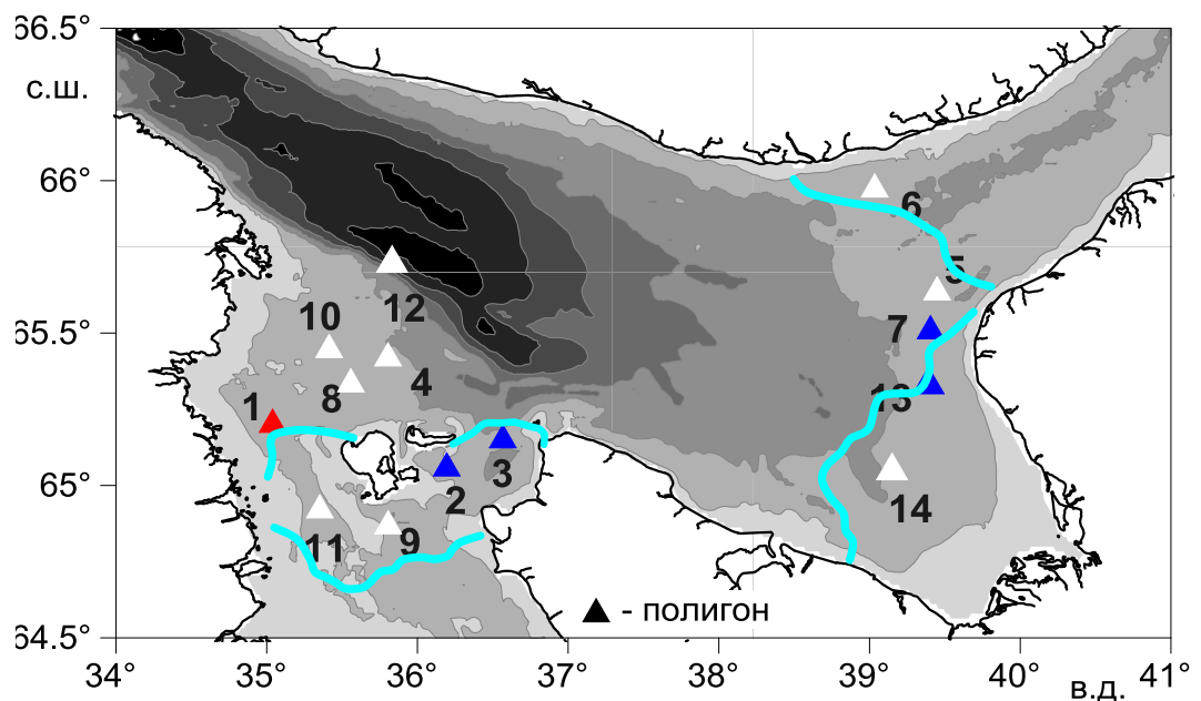
Рис. 5.4. Карта полигонов с оценками вклада внутренних волн в вертикальный обмен.
