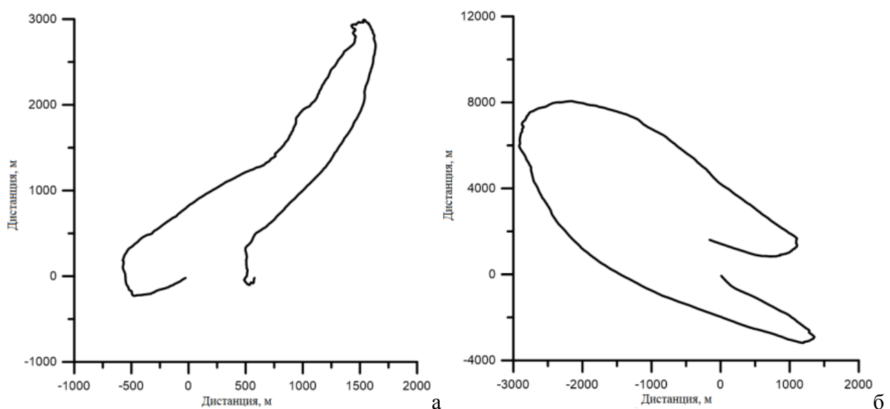
Рис. 2.15. Прогрессивные векторные диаграммы по данным, полученным с 08:23 по 20:47 24 июля 2012 г. на полигоне № 4 (а) и с 0:00 по 12:24 23 июля 2012 г. на полигоне № 3 (б) при
