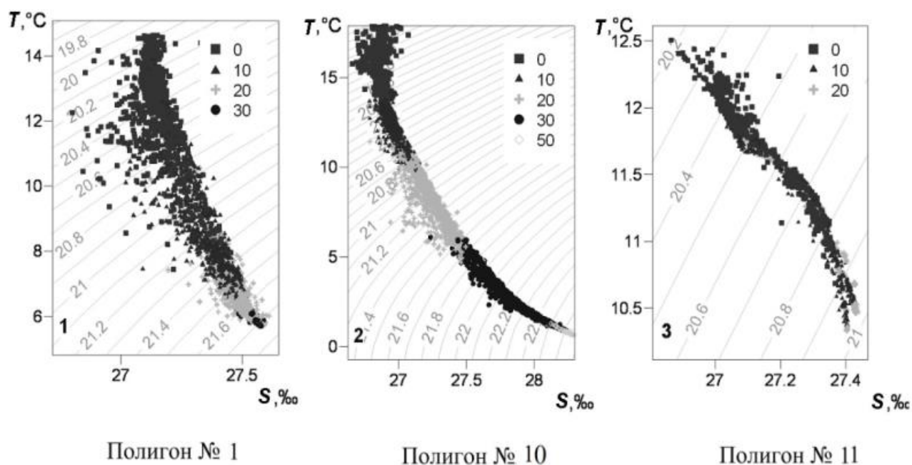
Рис. 2.2. T,S-кривые по данным наблюдений на полигонах (горизонты наблюдений обозначены на рисунке значками, соответствующие им глубины приведены в верхней правой части каждой кривой).
