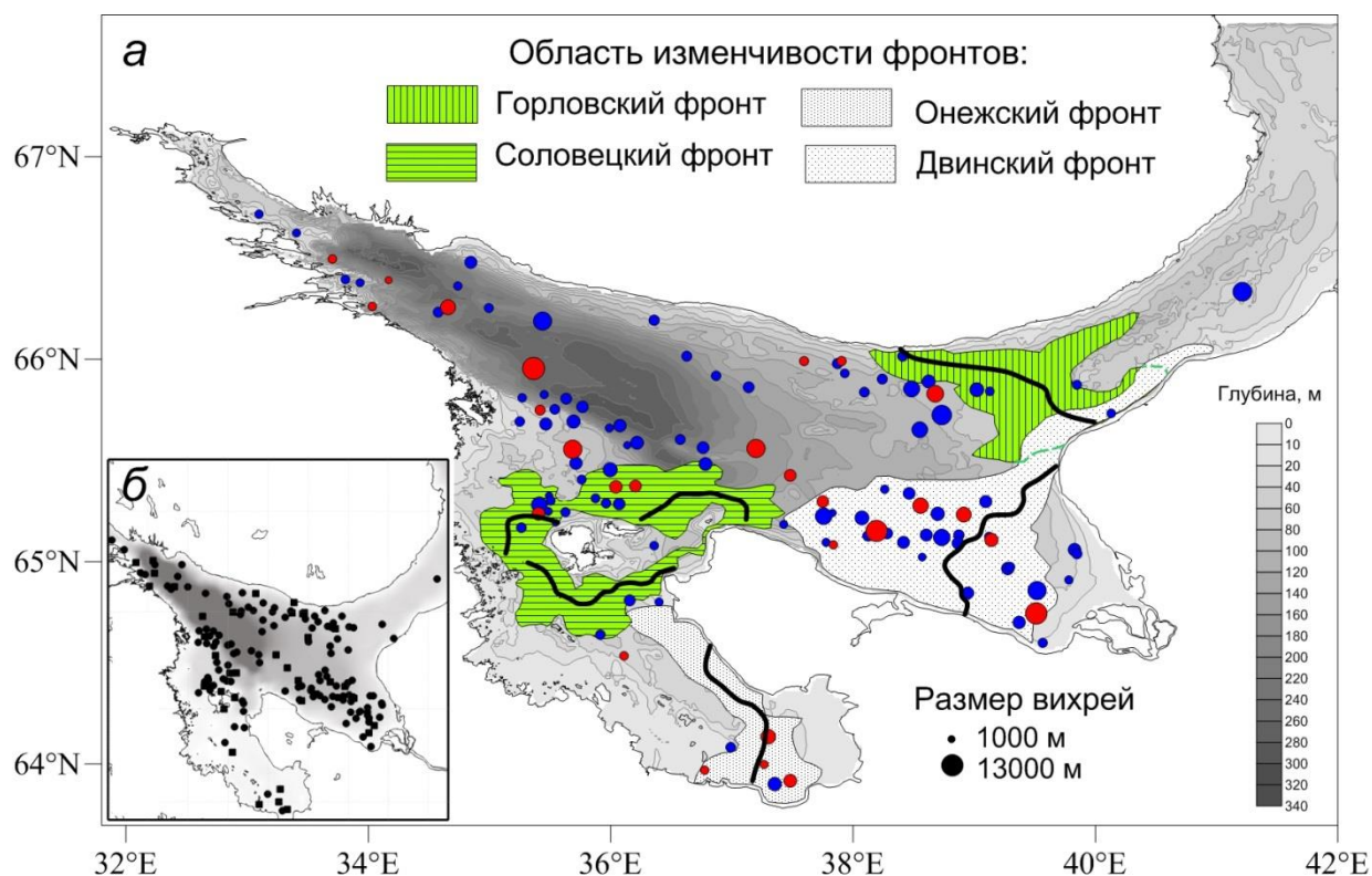
Рис. 4.14. Область изменчивости поверхностных фронтов, среднее за сезон положение фронтов и субмезомасштабные вихри в Белом море по спутниковым данным. а – композитная карта с
