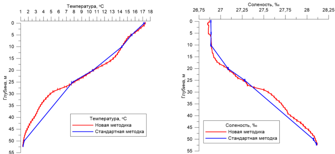
Рис. 2.10. Изменение с глубиной средних значений и стандартного отклонения температуры и солёности по данным сканирования CTD-90M на полигоне № 10 (Бассейн) 22.07.2011 г.
