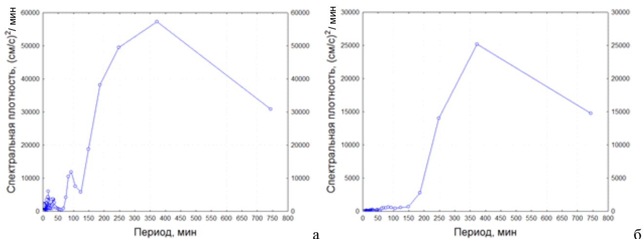
Рис. 2.16. Функции спектральной плотности с удаленным трендом ( M_2 ), по данным наблюдений за широтной составляющей скорости течения ( U ) на полигоне №1 на глубине 10 метров 18 июля 2012г (а) и на глубине 11 метров 27 июля 2011 г (б).
