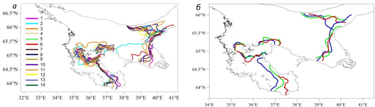
Рис. 4.7 Сезонная изменчивость положения фронтальных разделов на поверхности Белого моря: а – положения для каждой из 14-ти декад; б – положения по среднемесячным данным за июнь (синяя линия), июль (зеленая линия) и август (красная линия).
