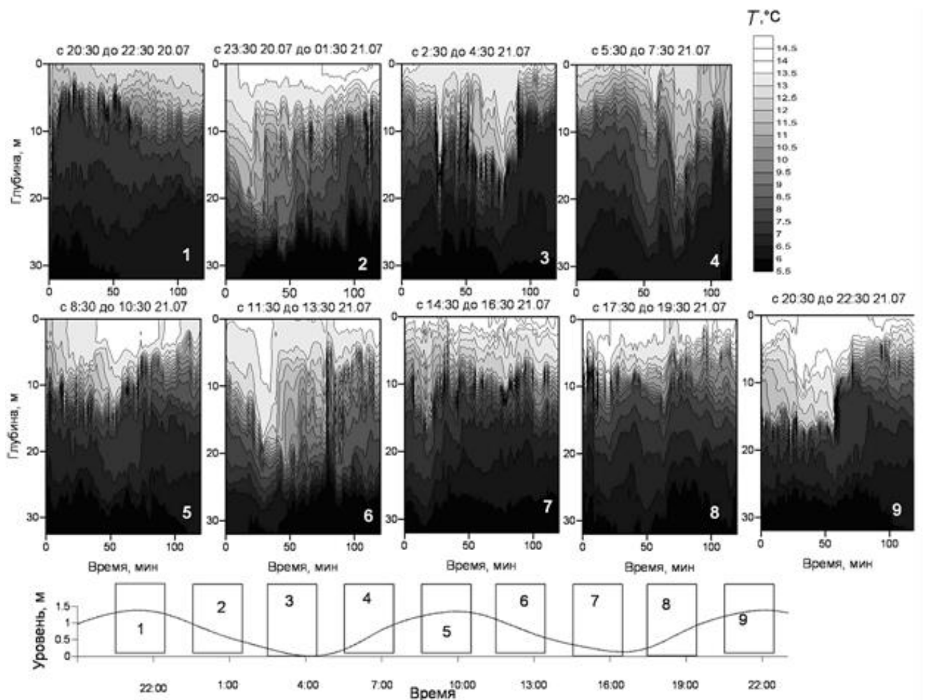
Рис. 2.6. . Временная изменчивость температуры по данным сканирования CTD - 90М на полигоне № 1 (мористая часть пролива Западная Соловецкая салма) с 20:30 20.07.2011г. до
