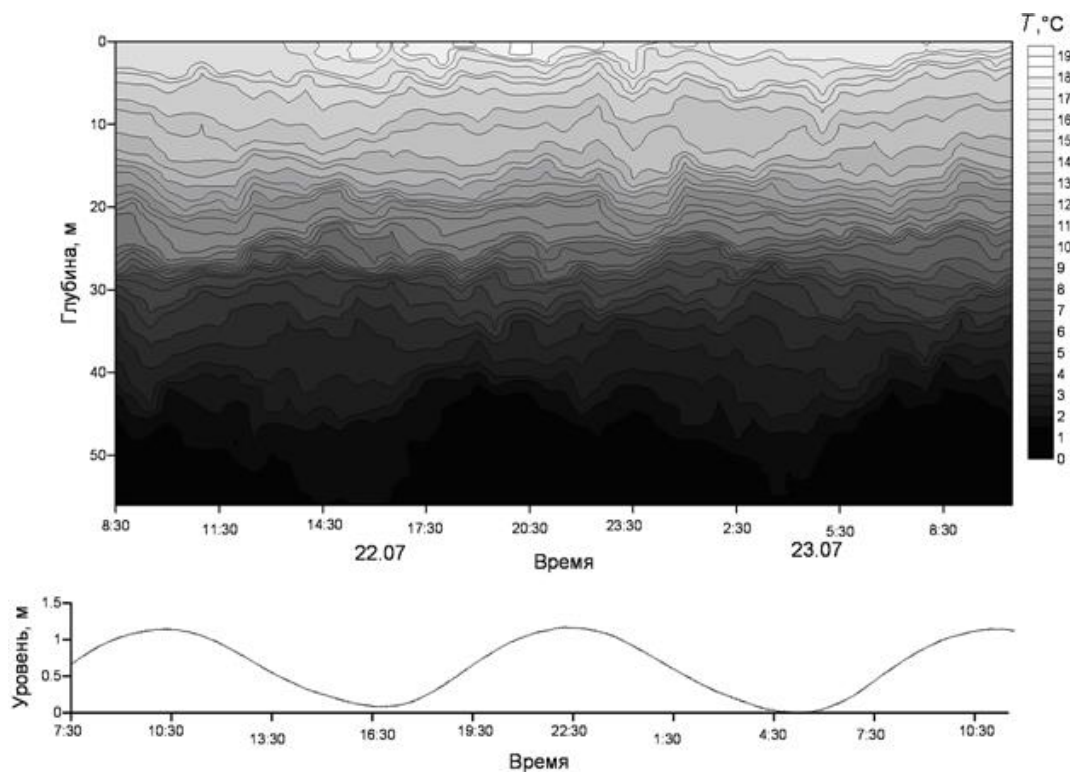
Рис. 2.4. Временная изменчивость температуры по данным измерений CTD - 90М и колебания уровня на полигоне № 10 (Бассейн Белого моря) с 8.30 22.07.2011 г. до 10.30 23.07.2011 г.
