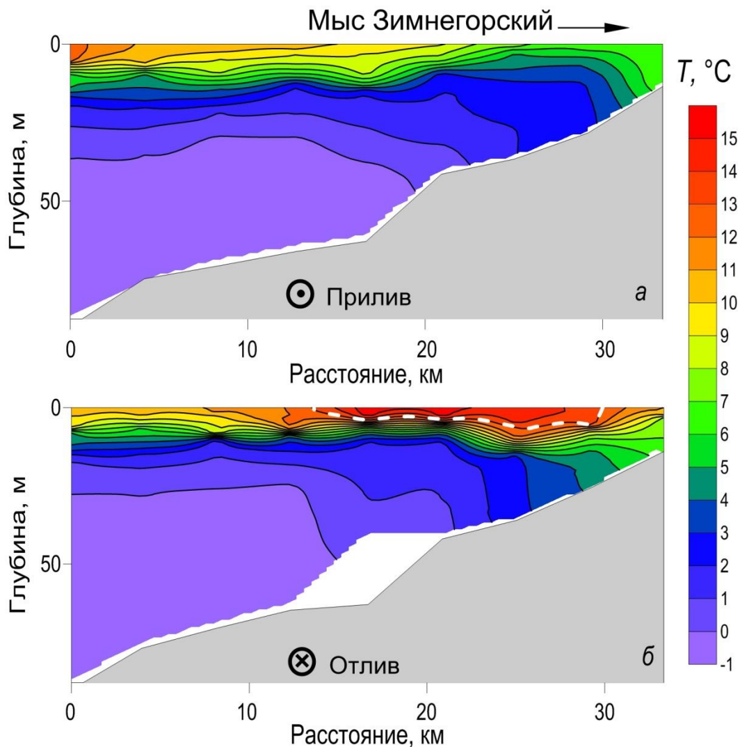
Рис. 4.11. Распределение температуры на разрезе в Двинском заливе, выполненном 24.07.2014г. (а) и 25-26.07.2014 г. (б).
