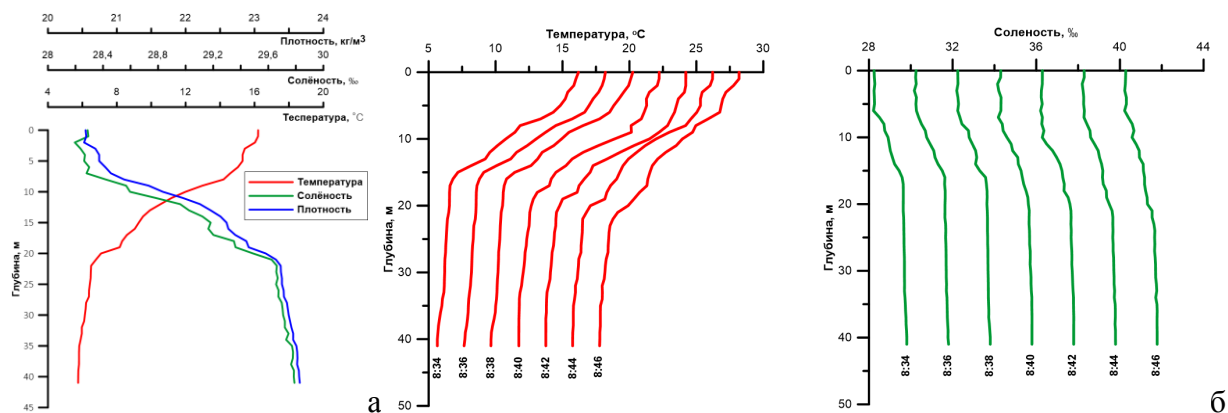
Рис. 2.17. Характерные профили температуры, солености и условной плотности для полигона №1 июля 2012 года (а) и серии профилей температуры и солености, записанные 18 июля 2012 года (б)
