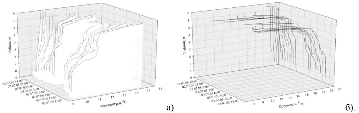
Рис. 1.6. Временной ход вертикального распределения температуры и солёности в Онежском заливе. По данным измерений ИВПС КарНЦ РАН летом 2005 г. [Филатов и Тержевик, 2007].
