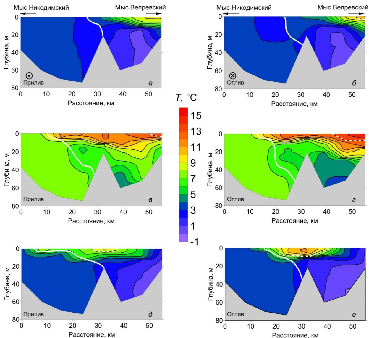
Рис. 4.9. Распределение температуры на разрезах, выполненных в зоне Горловского фронта в июне 2014 г. (а и б), августе 2012 г. (в и г), июле 2009 г. (д и е). Фрагменты а, в, д соответствуют течениям в прилив (течения направлены из пролива), а фрагменты б, г, е – в отлив.
