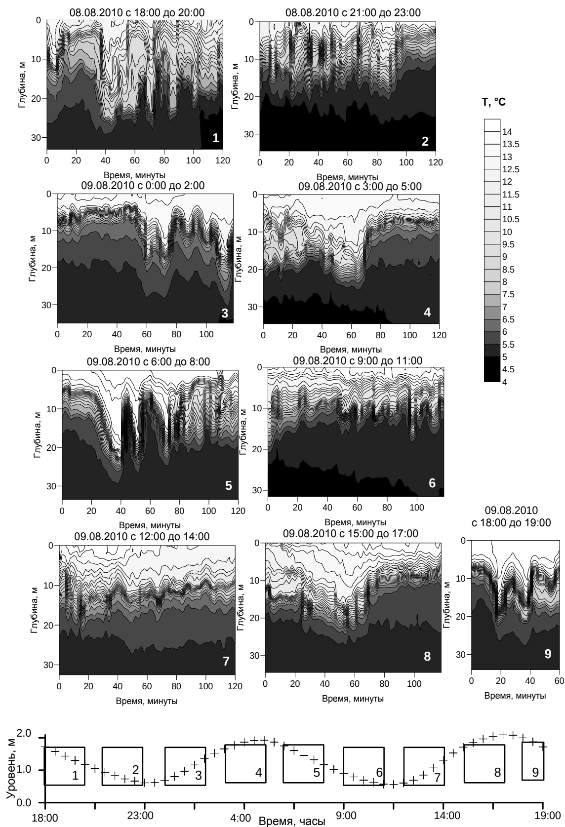
Рис.3.2. Временная изменчивость температуры по данным сканирования на суточной станции с 18:00 8.08.2010 до 19:00 9.08.2010 на южной границе полигона и колебания уровня по
