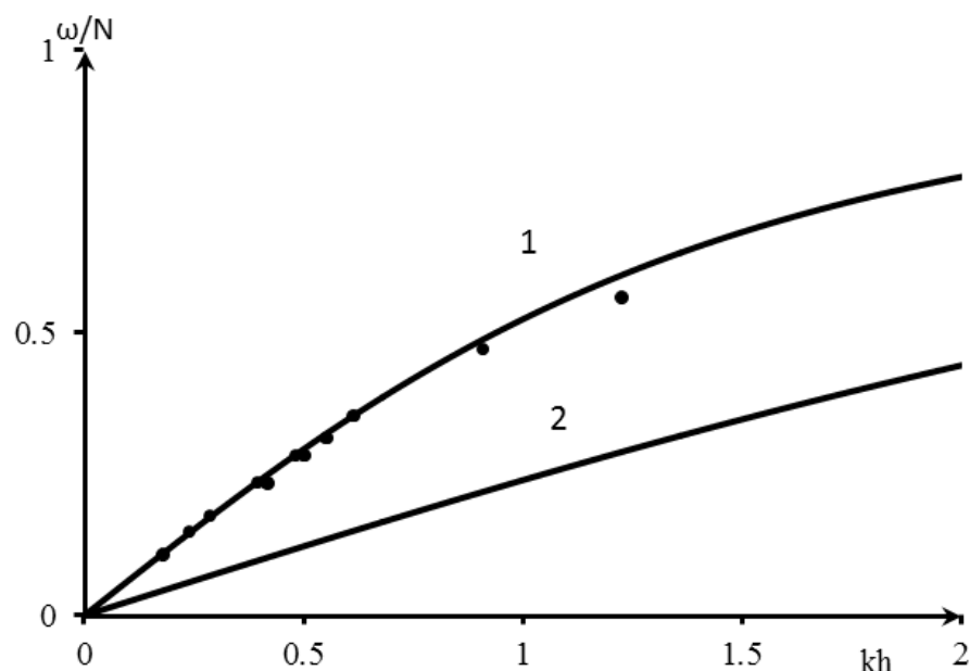
Рис.3.5. Дисперсионные кривые для первой (1) и второй (2) моды внутренних волн для случая постоянного профиля плотности (линии) и экспериментальные оценки дисперсионного соотношения (точки) построенные по данным наблюдений на полигоне №1.
