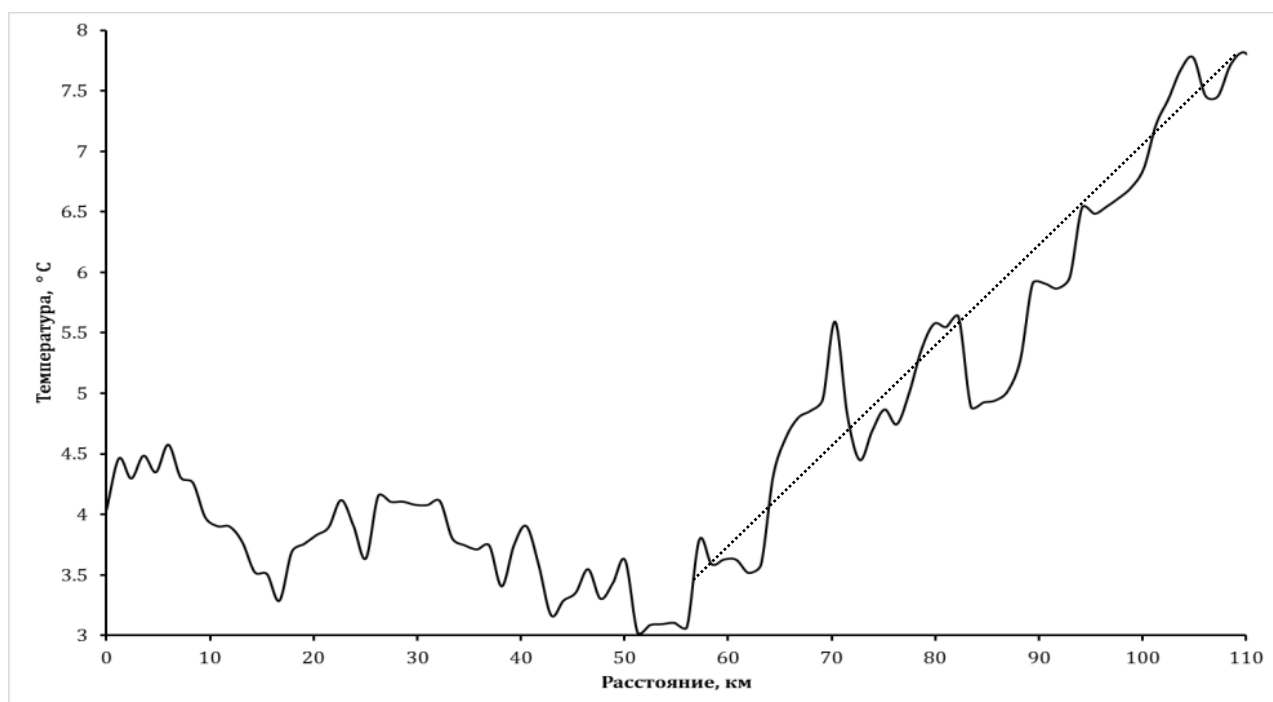
Рис.4.10. Распределение ТПМ на разрезе G3 через фронтальную зону Горла по данным за первую декаду июля 2010 года.
