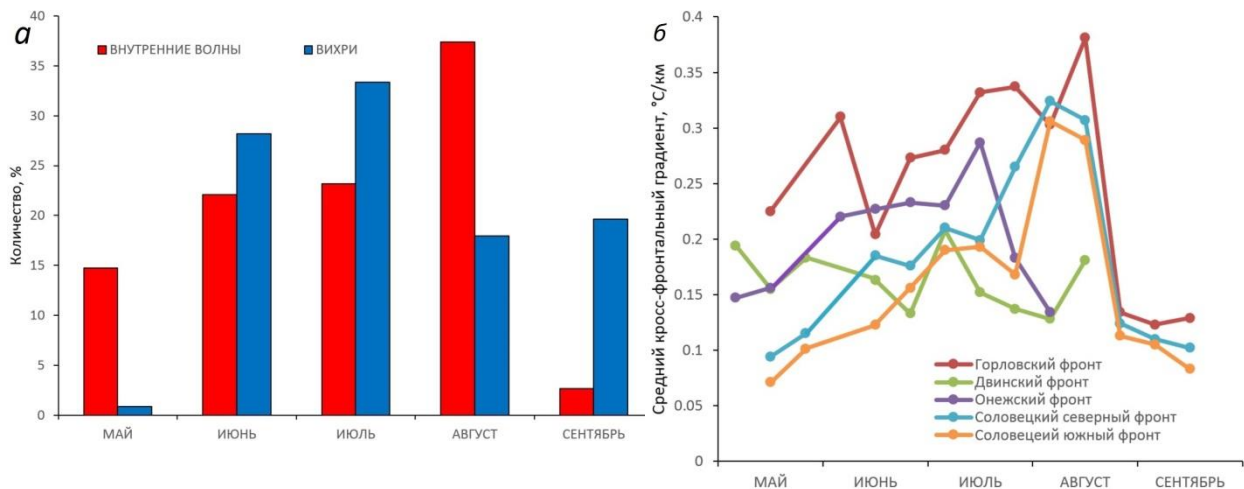
Рис. 4.16. Сезонный ход поверхностных проявлений вихрей, короткопериодных внутренних волн и градиентов ТПМ на фронтах в Белом море по спутниковым данным 2010 г.: а – относительное количество вихрей и волн; б – средний кросс-фронтальный градиент ТПМ по декадным оценкам.
