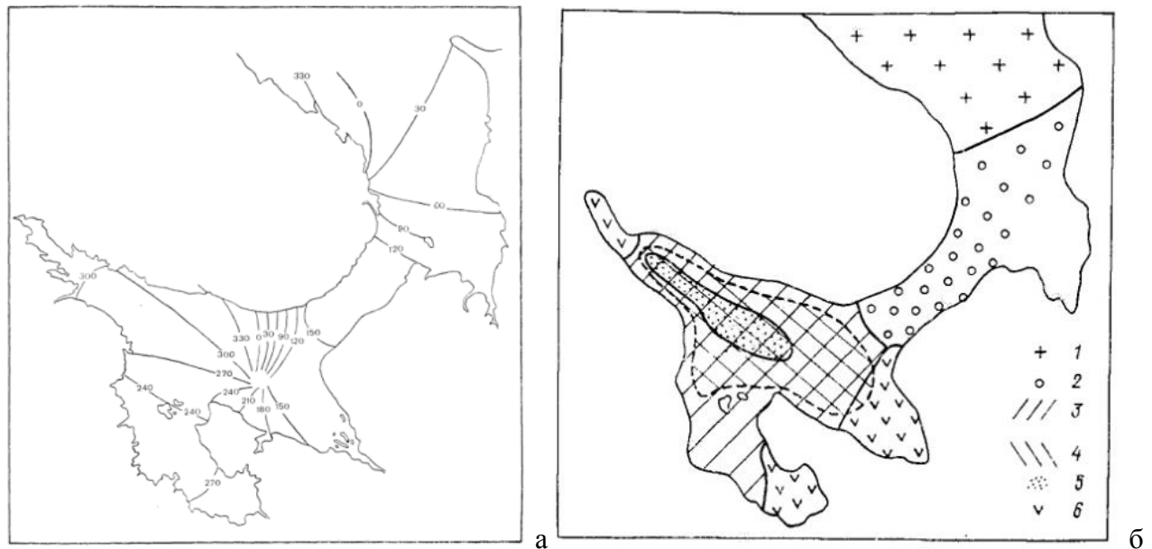
Рис. 1.3. Карта а) изофаз приливных течений M_2 , б) распределения водных масс летом 1 – баренцевоморская; 2 – водная масса Горла; 3 – поверхностная водная масса Бассейна; 4 – промежуточная; 5 – глубинная водная масса бассейна; 6 – распресненные воды заливов [Гидрометеорология..., 1991].
