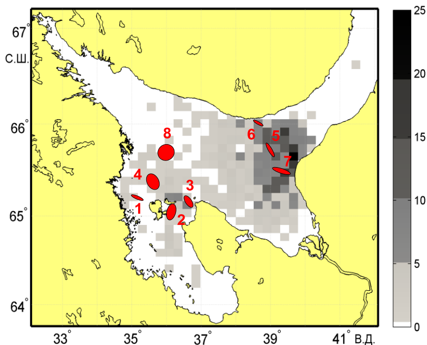
Рис. 5.2. Эллипсы горизонтального турбулентного обмена (обозначены красным) с номерами советующих полигонов, выполненных в июле – августе 2012 года, совмещенные с частотой встречаемости проявлений короткопериодных внутренних волн (обозначены серым) по данным
