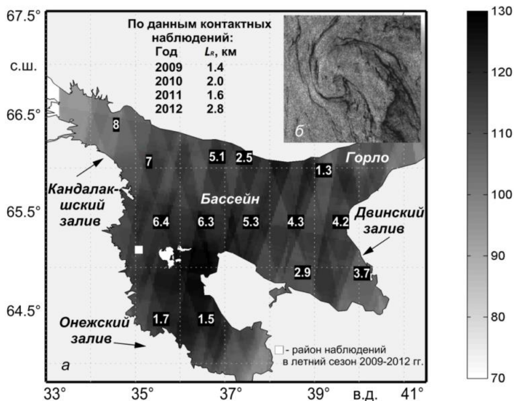
Рис. 4.1. Карта (а) покрытия акватории Белого моря РЛИ за теплый период 2009 - 2012 гг. Белыми цифрами на карте показаны значения бароклинного радиуса Россби (в км) по климатическим данным за август, в таблице – значения радиуса по данным наблюдений в районе, обозначенном белым квадратом. На врезке (б) представлен фрагмент РСА снимка Envisat ASAR от 04.08.2010 (08:23 UTC), относящийся к Бассейну Белого моря с примером проявления вихревой структуры. © CSA
