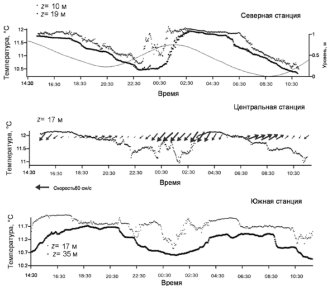
Рис. 2.7. Вариации температуры воды на южной (по CTD-90M, ADP Sontek-500), центральной (по «Вектор-2») и северной станциях (по «JFE Ales»), скорости и направления течения на центральной станции и колебания уровня (по ADCP WHS 300) на северной станции по данным наблюдений на полигоне № 3 (узкая часть пролива Западная Соловецкая салма) с 14:30 24.07.2011 г. до 11:00 25.07.2011 г.
