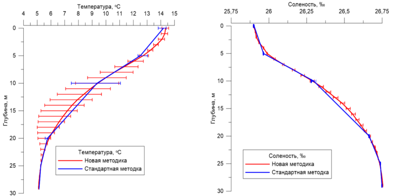
Рис. 2.9. Изменение с глубиной средних значений и стандартного отклонения температуры и солёности по данным сканирования CTD-90M на полигоне № 1 (мористая часть пролива Западная Соловецкая салма) 9.08.2010 г.
