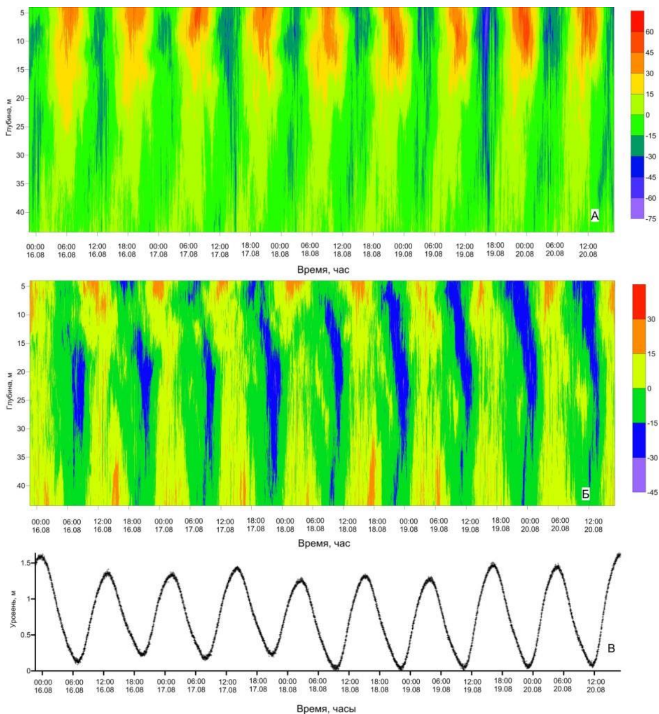
Рис. 2.13. Временная изменчивость скорости и направления течения: скорость вдоль оси север-юг (а), восток-запад (б) и колебания уровня (в) по данным акустического профилографа ADCP WHS -300, установленного на северной границе полигона № 1 с 15 по 20 августа 2013 г.
