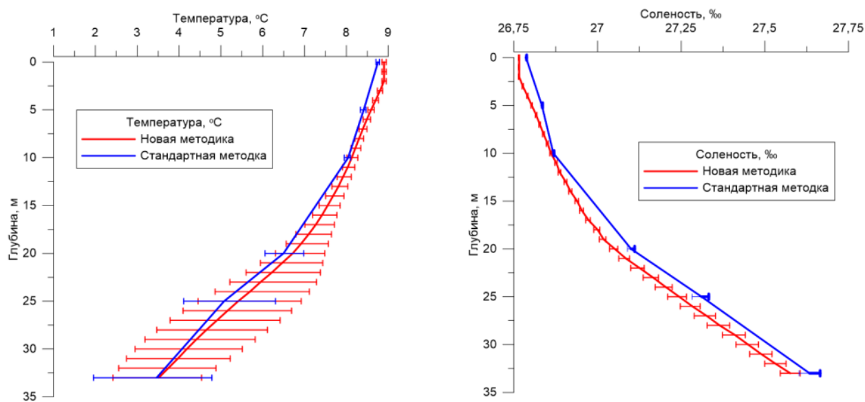
Рис. 2.11. Изменение с глубиной средних значений и стандартного отклонения температуры и солёности по данным сканирования CTD-90M на полигоне № 3 (Восточная Соловецкая салма) 23.07.2014 г.
