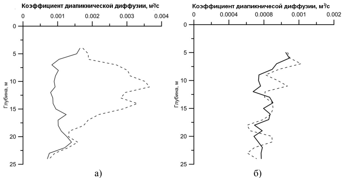
Рис. 5.3. Вертикальная изменчивость за приливной цикл коэффициента диапикнической диффузии по данным наблюдений на полигоне № 1 в 2011 году (а) и полигоне № 4 в 2012 году (б). Жирной линией показаны результаты расчетов, выполненных по данным с интервалом осреднения 2 часа, пунктирной линией – 2 минуты.
