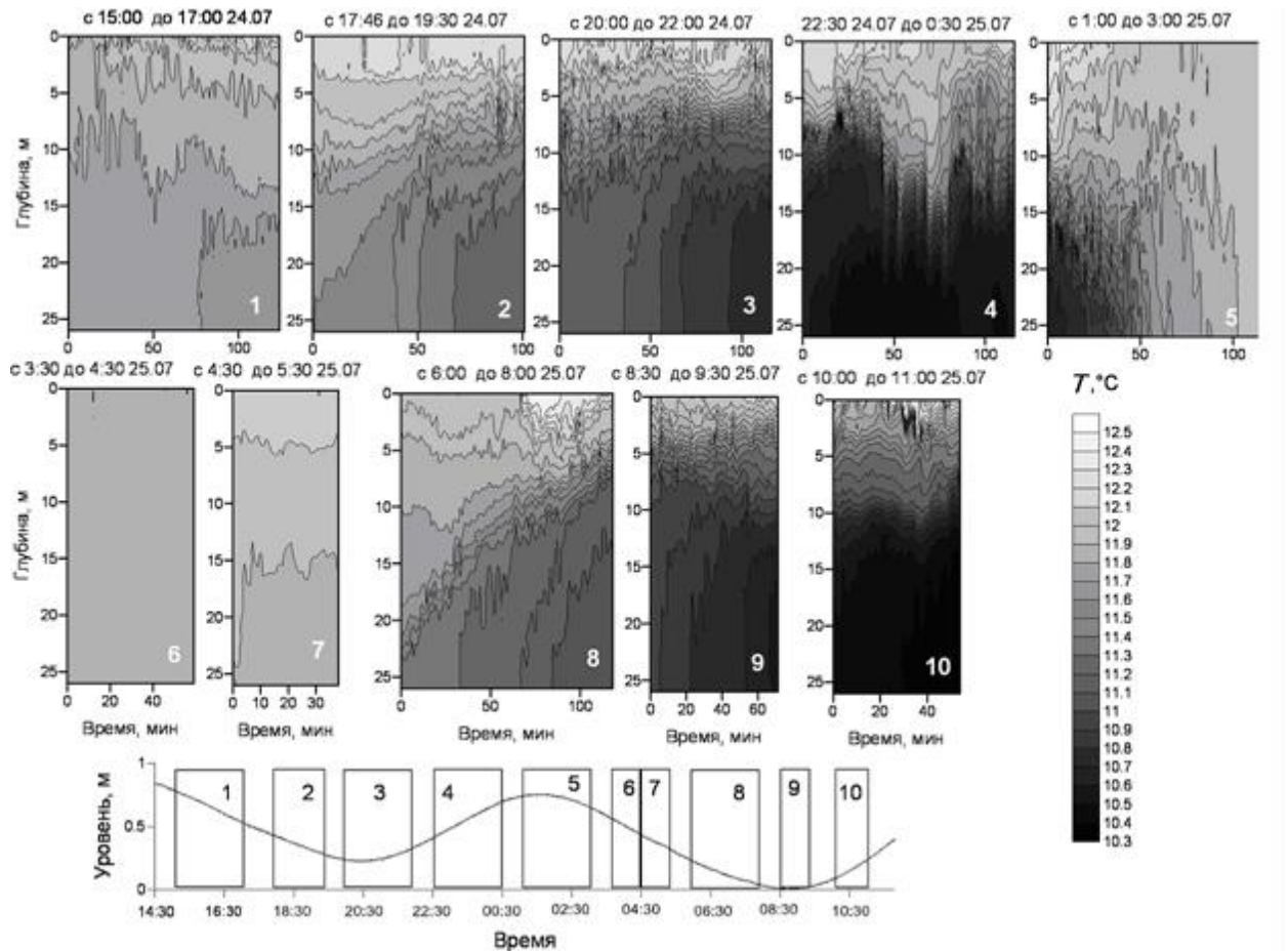
Рис. 2.8. Временная изменчивость температуры по данным сканирования CTD - зондом на полигоне № 11 (узкая часть пролива Западная Соловецкая салма) с 15:00 24.07.2011 г. до 11:30 25.07.2011 г. и колебания уровня (прямоугольниками с номерами показаны периоды сканирований)
