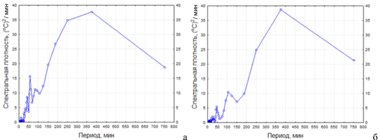
Рис. 2.12. Функция спектральной плотности с удаленным трендом ( M_2 ) по данным наблюдений за температурой на буйковой станции с помощью прибора JFE Alec, установленного на горизонте 12 метров (а) и 9 метров (б) на полигоне № 4 (Бассейн) 24 июля 2012 г.
