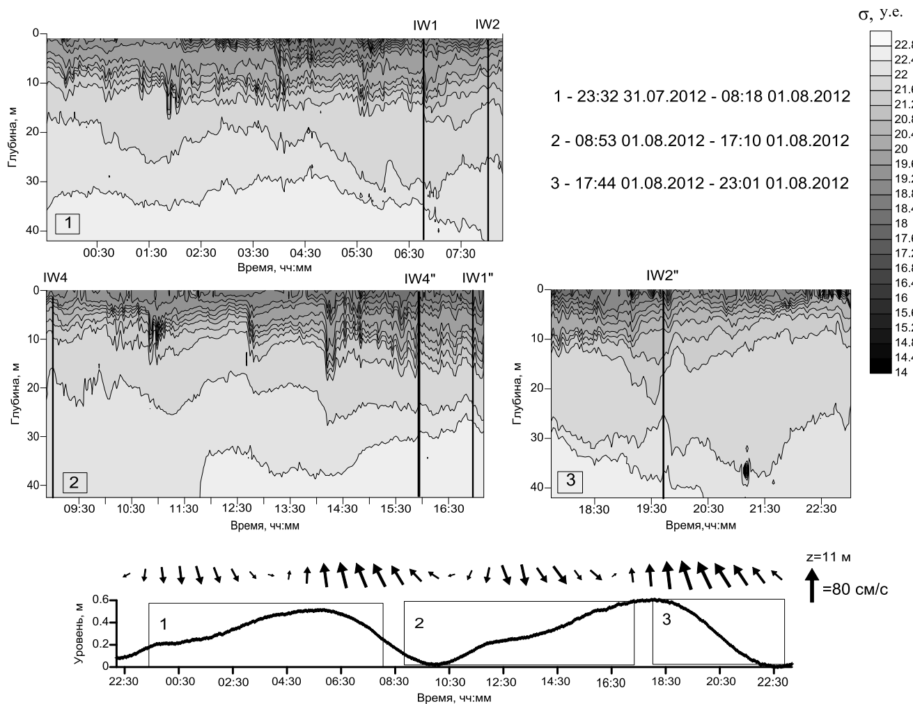
Рис. 3.9. Временная изменчивость вертикального распределения плотности по данным сканирований СТД-зондом, скорости течения на горизонте 11 м и колебаний уровня моря по данным ADP SonTek-500 с 22.30 31.07.2012 г. до 23.30 1.08.2012 г. Нижний ряд прямоугольников с номерами на графике хода уровня показывает периоды сканирований, которые указаны на рисунке. На графике сканирований обозначены моменты времени прохождения через точку наблюдения сигнатур, идентифицируемых по данным RADARSAT-1 (IW1, IW2 IW4) и RADARSAT-2 (IW1'', IW2'', IW4'') за 1.08.2012 г.
