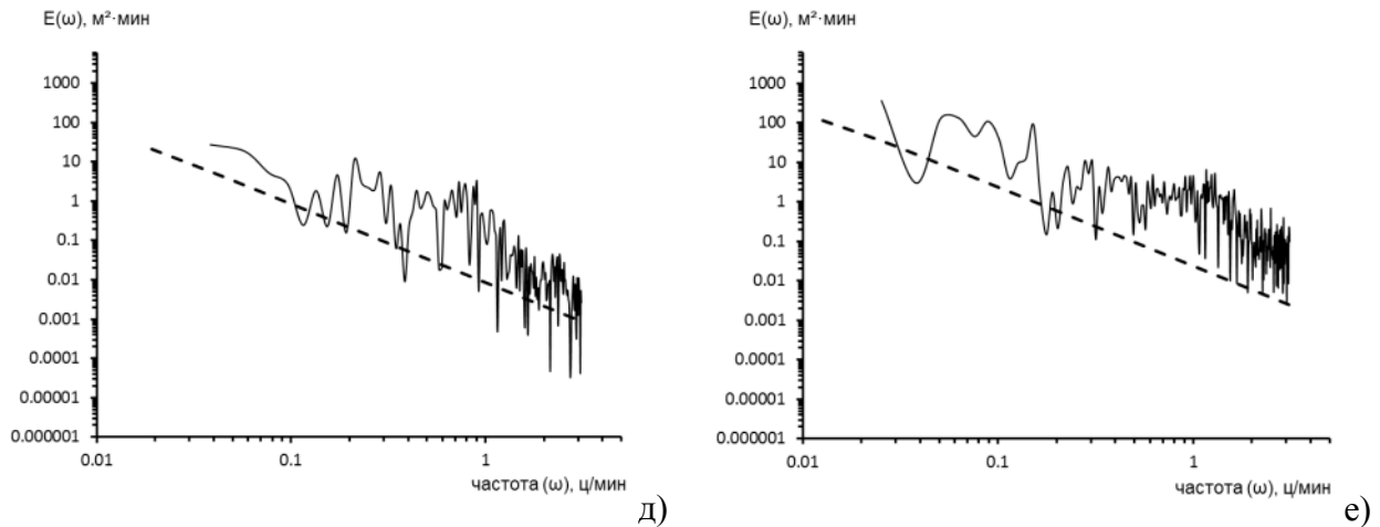
Рис. 3.3 Временные спектры вертикальных смещений термоклина (пикноклина) по данным на полигоне № 1 (а), № 2 (б), № 3 (в) № 4 (г), № 5 (г), № 7(д) в 2012 г. Спектры, построенные по данным измерений, обозначены сплошной линией. Пунктиром показан спектр Гарретта – Манка.
