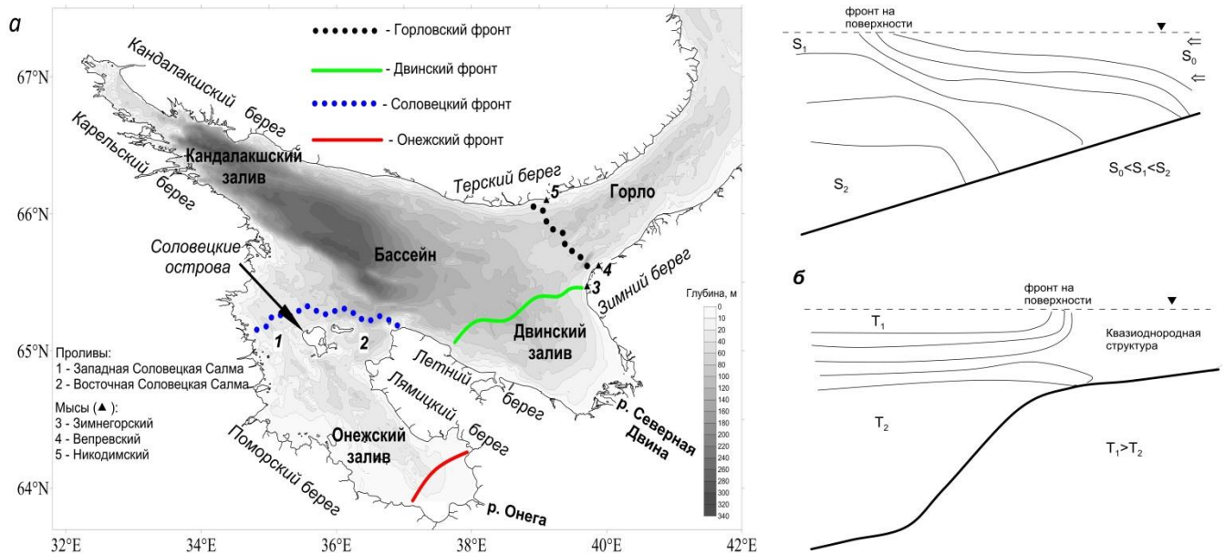
Рис. 1.4. Белое море и его основные гидрологические фронты. а - Карта Белого моря с положением фронтов [Пантюлин, 2012] и б – геометрия фронтальных разделов стокового (сверху) и шельфового (снизу) типа. S_0, S_1, S_2 – соленость, T_1, T_2 – температура.
